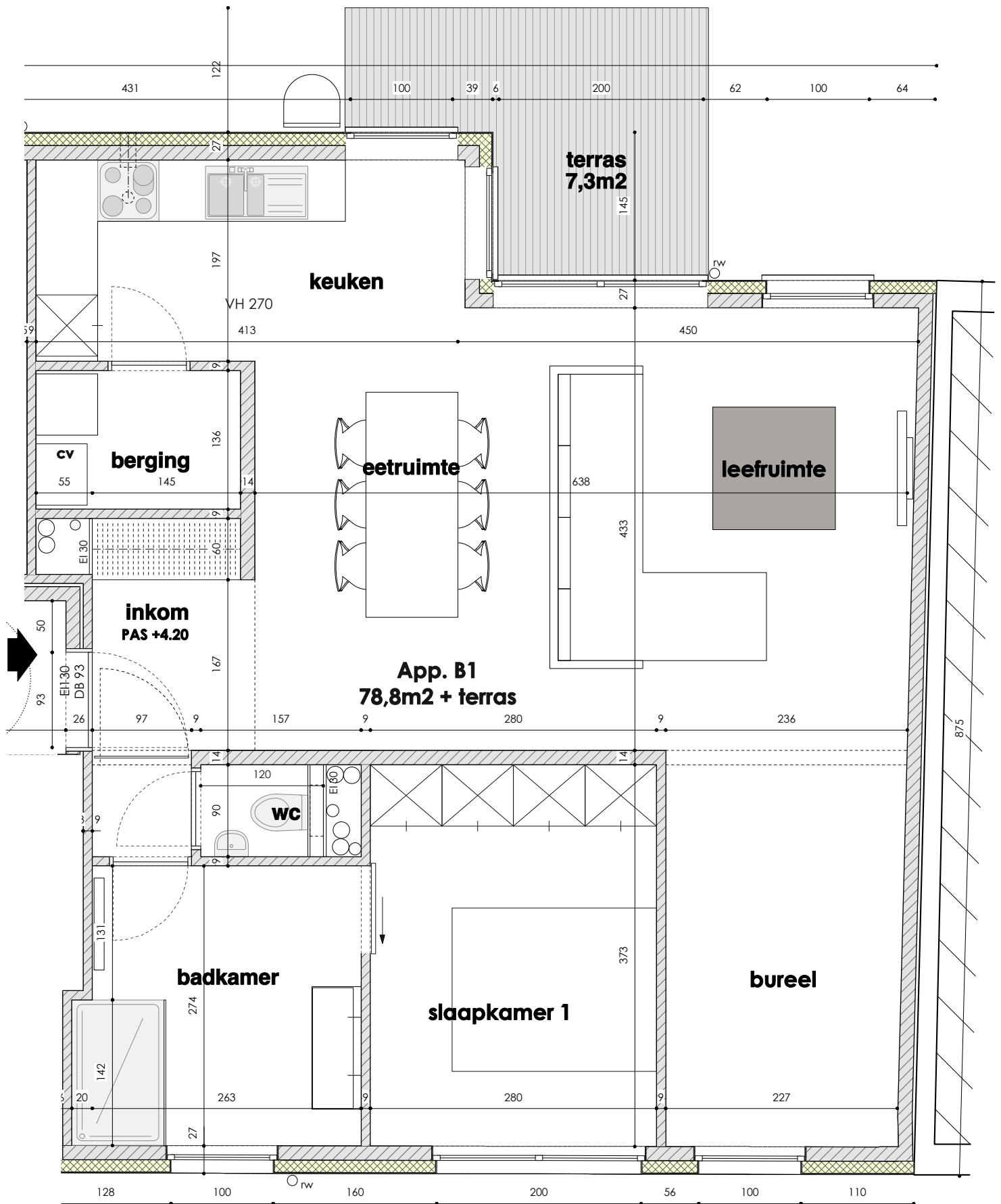
GRONDPLAN B1 1/50
