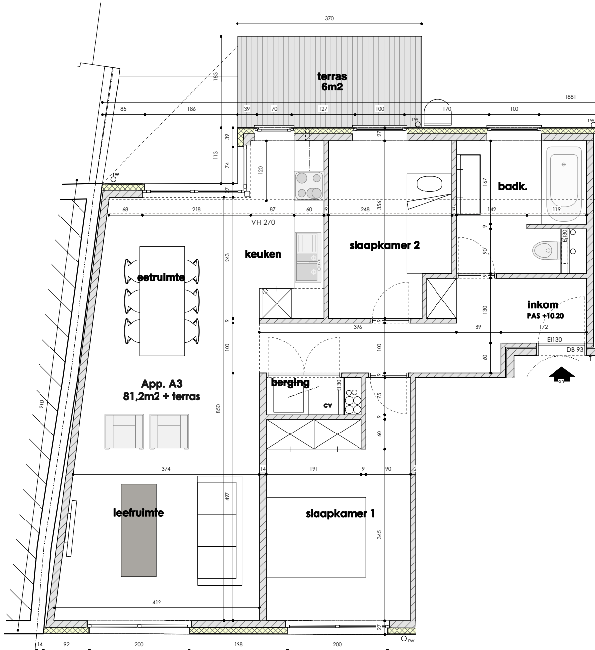
GRONDPLAN A3 1/75
