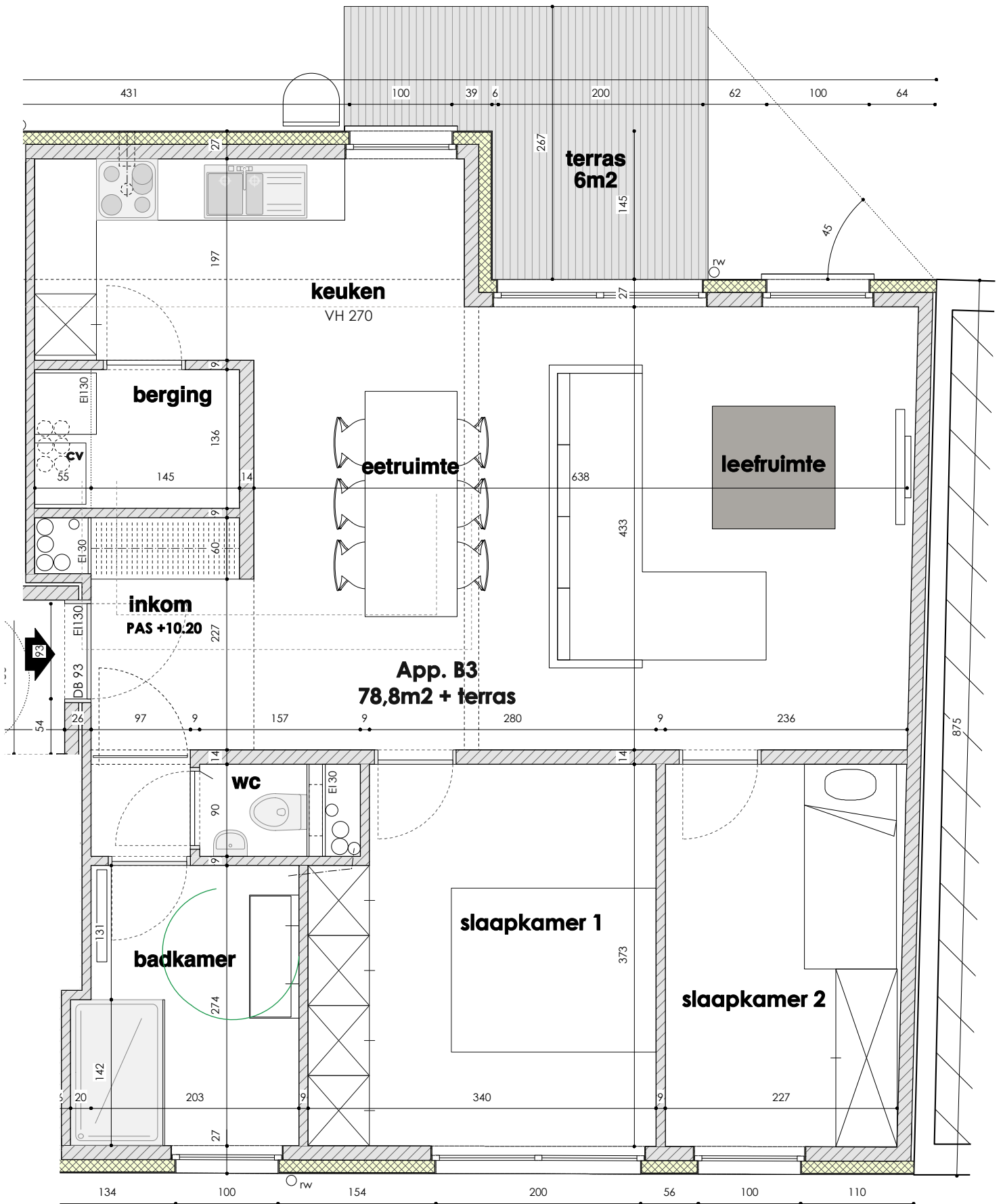
GRONDPLAN B3 1/50
